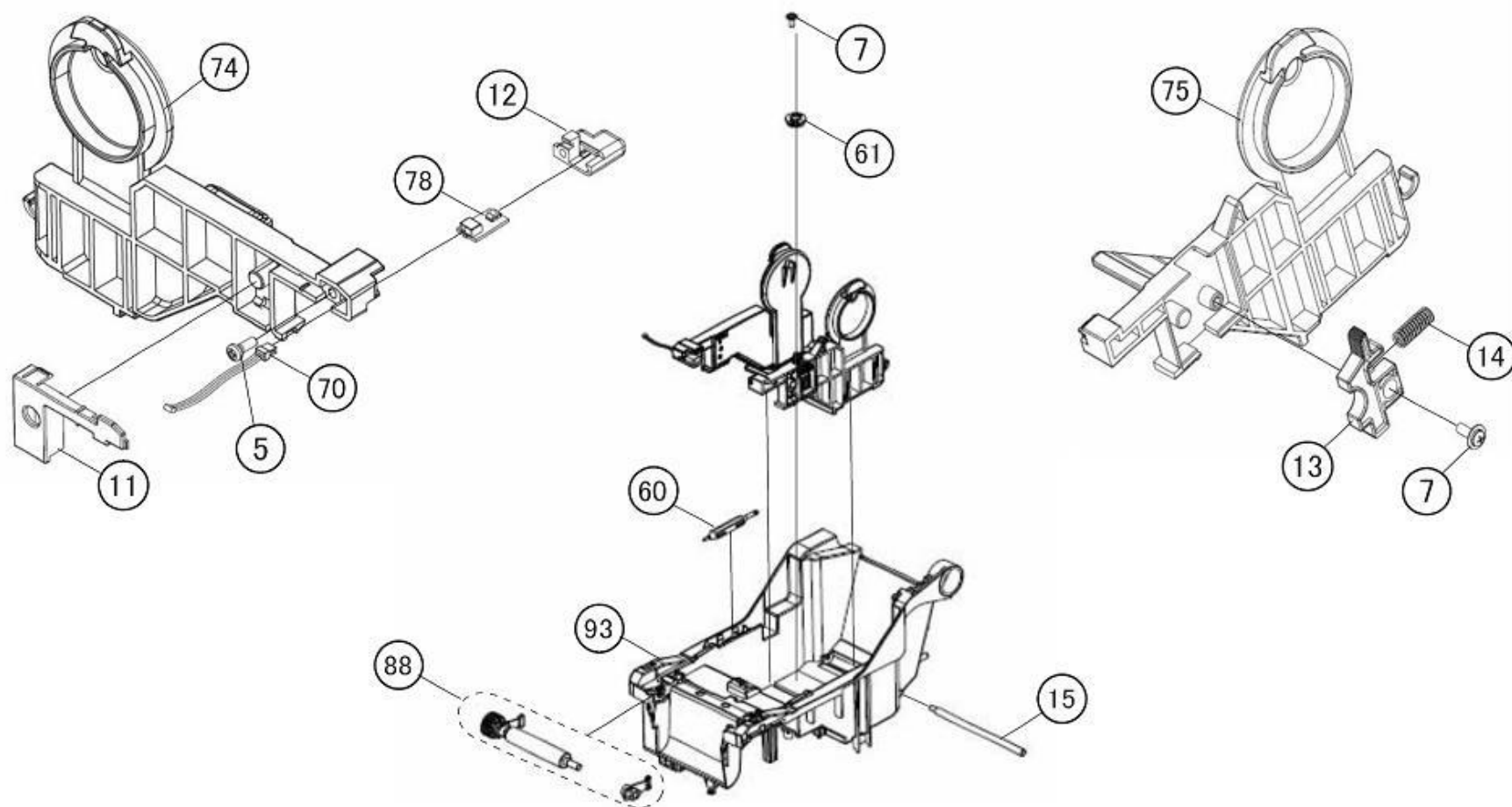
DESCRIPTION Fig04-ASSY(04)
